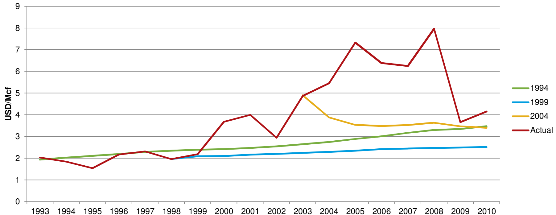
U.S. EIA prognozuota ir reali dujų kaina 1994, 1999, 2004 m. prognozės
