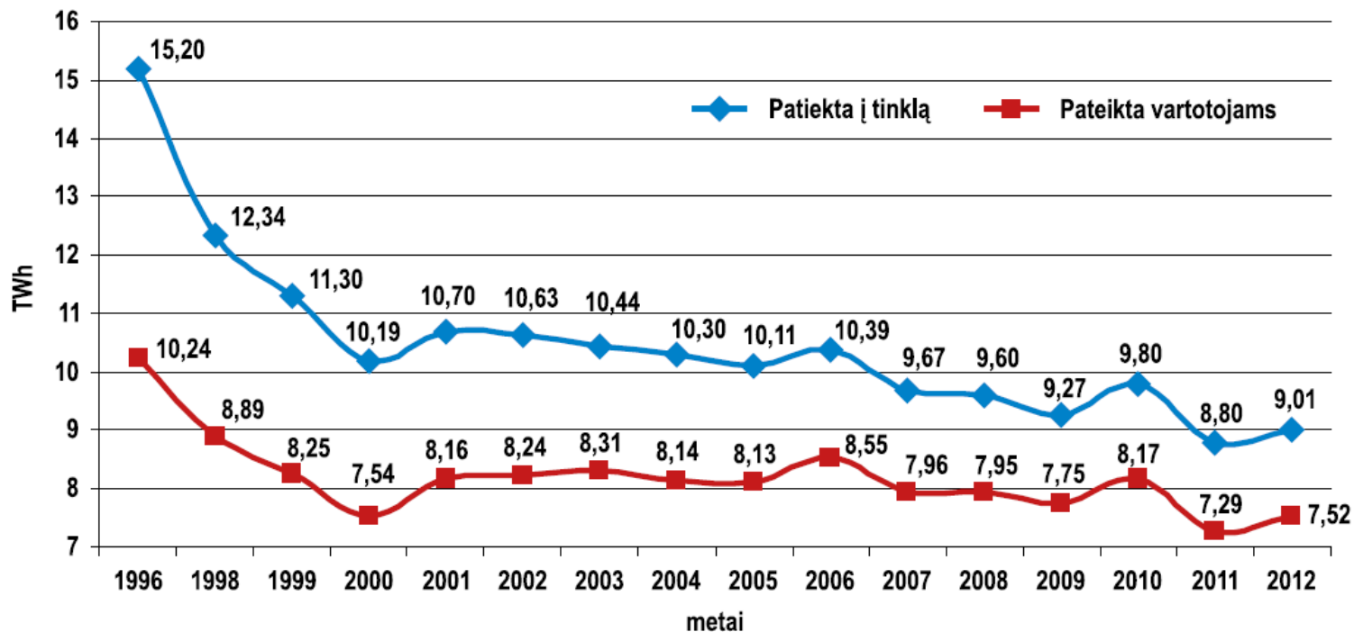
Šilumos energijos gamybos balansas Lietuvoje 1996–2012
